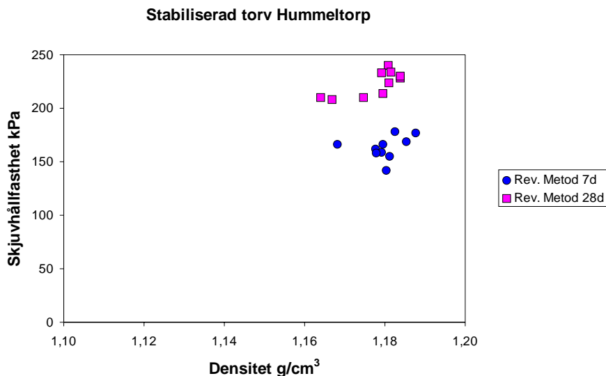
Figur 7. Resultat från provtryckning av provkroppar tillverkade med den reviderade metoden.
